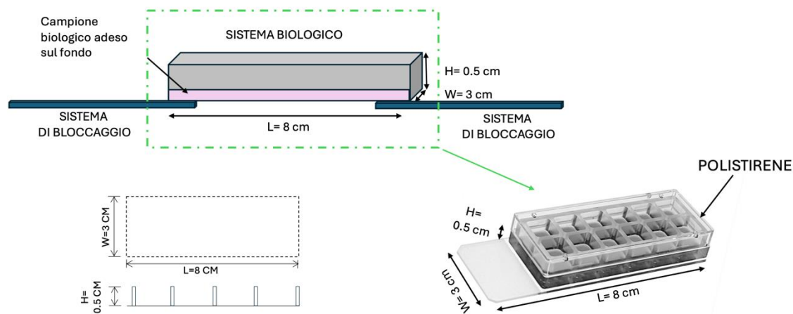
Figura 1. Schema rappresentante il volume (8 cm (l), 3 cm (w), 0.5 cm (h)) contenente il sistema biologico in cui il campo magnetico generato deve essere spazialmente uniforme. Lo schema include anche l'holder che deve essere incluso nella fornitura dove alloggiare nella posizione opportuna il sistema biologico.
